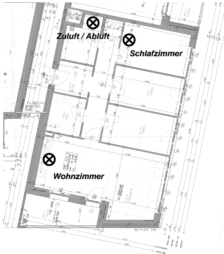
Abbildung 5: Planskizze der gemessenen Wohnung im Passivhaus Kammelweg mit Angabe der Positionen der Sensoren (Kreise mit Kreuz). Norden ist oben auf dem Bild.
