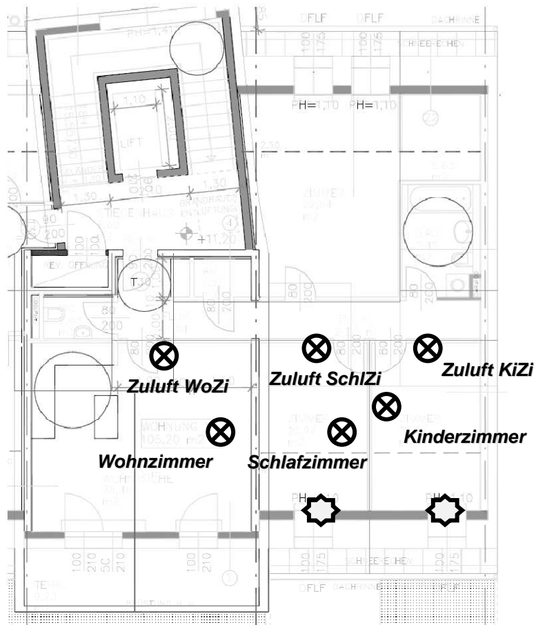
Abbildung 6: Planskizze der gemessenen Wohnung im Passivhaus Utendorfgasse mit Angabe der Positionen der Sensoren (Kreise mit Kreuz = Temperatur und Luftfeuchtigkeit, Acht-Stern = Fensteröffnung). Norden ist oben auf dem Bild.
