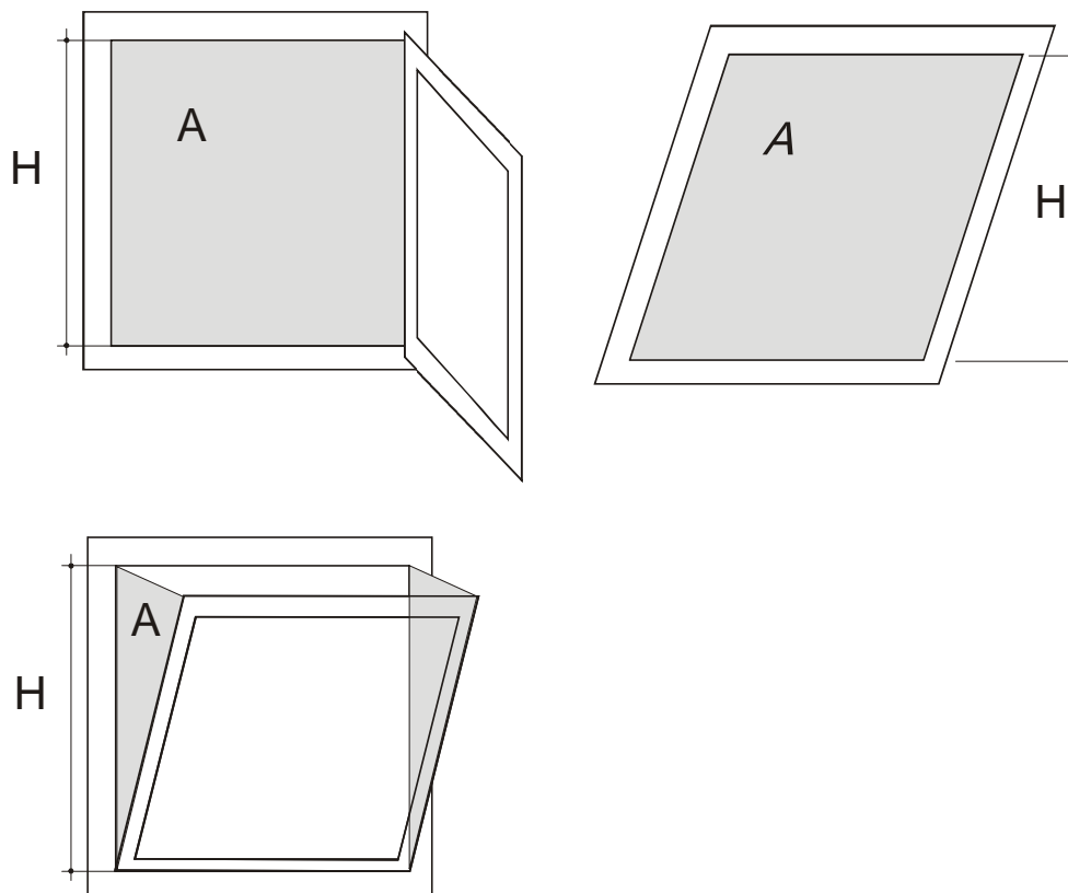
Abbildung 31: Definition von A und H für verschiedene Konfigurationen von öffnenbaren FensterTüren
