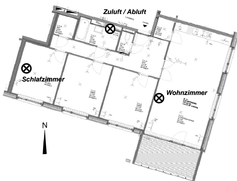
Abbildung 1: Planskizze der gemessenen Wohnung im Passivhaus Mühlweg mit Angabe der Positionen der Sensoren (Kreise mit Kreuz).
